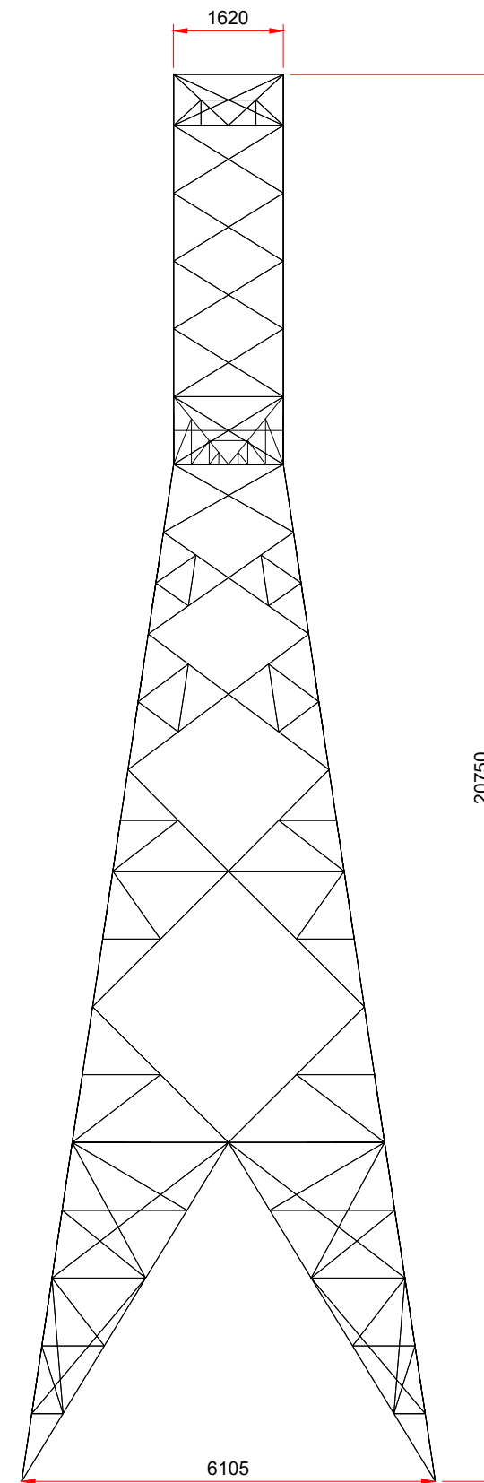
SIDE ELEVATION SCALE: 1:100
