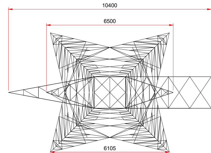
PLAN VIEW SCALE: 1:100
