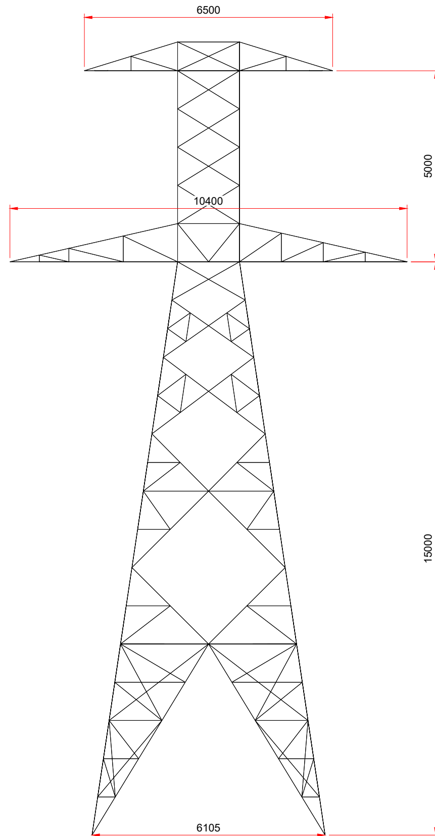
FRONT ELEVATION SCALE: 1:100
